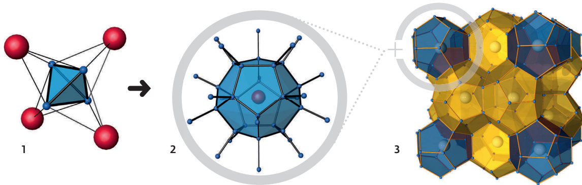
Konstruktion chemischer Käfige: Die molekularen Bausteine (1) der Clathrate bestehen aus Silizium (blau) und einem Metall (rot) wie Natrium, Kalium oder Barium. Daraus bilden sich Siliziumpolyeder (2), welche die Metallatome wie Käfige umschließen. Die Polyeder stapeln sich zu einem voluminösen Gerüst (3).
