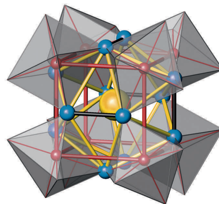
Blick in ein Skutterudit mit Füllung: Die roten Kugeln stehen für Kobalt-, Rhodium- oder Iridiumatome, die blauen für Phosphor, Arsen oder Antimon. In den Hohlräumen des Gerüsts finden Calcium- oder Bariumatome (gelb) Platz. In Grau sind oktaedrische Strukturelemente angedeutet.
